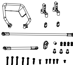
500405649 Umbauset Allradlenkung 4WD Steeringkit
