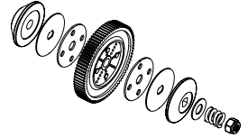
500405615 Maingear/slipperclutch Set Rutschkupplung-/Zahnrad Set
