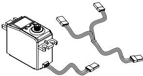
500502046 Servo f. 4WD Lenkung inkl. V-Kabel / Servo f. 4WD Steering incl. V-cable
