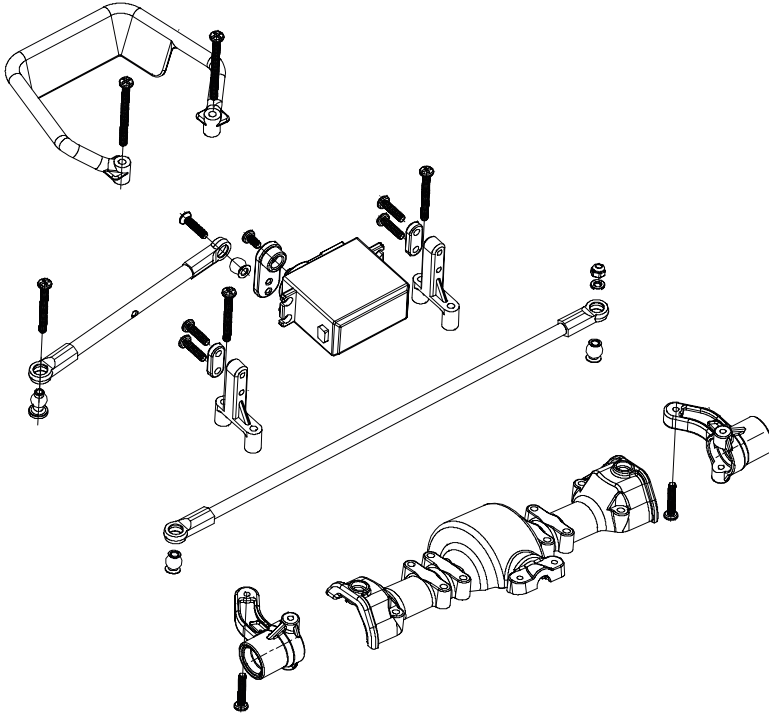
500502046 Servo f. 4WD Lenkung inkl. V-Kabel / Servo f. 4WD Steering incl. V-cable
