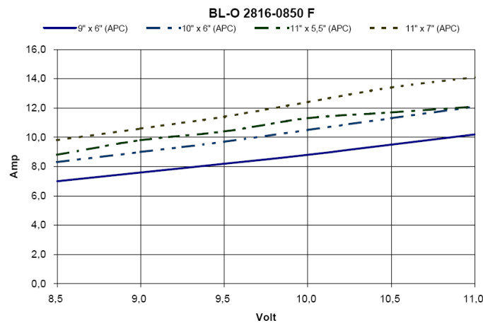
BL-O 2816-0850 F Strom über Spannung mit versch. Luftschrauben
