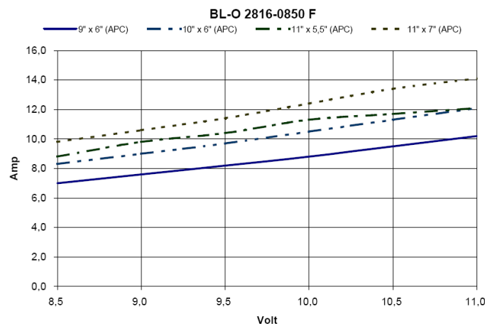
PERMAX BL-O 2816-0850 F courant/tension avec différentes hélices
