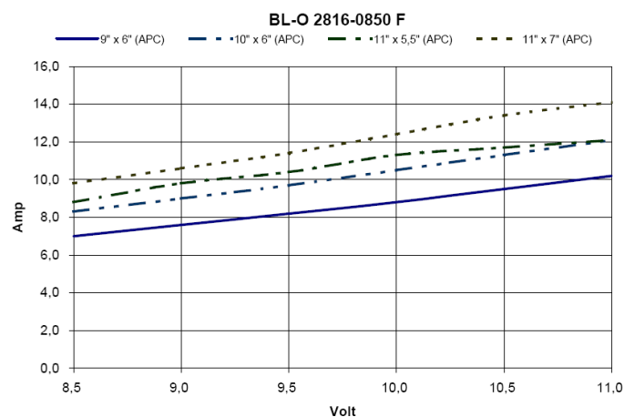
PERMAX BL-O 2816-0850 F Corrente e tensione con eliche diverse
