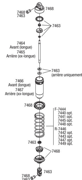
D. Installation/enlèvement du piston
