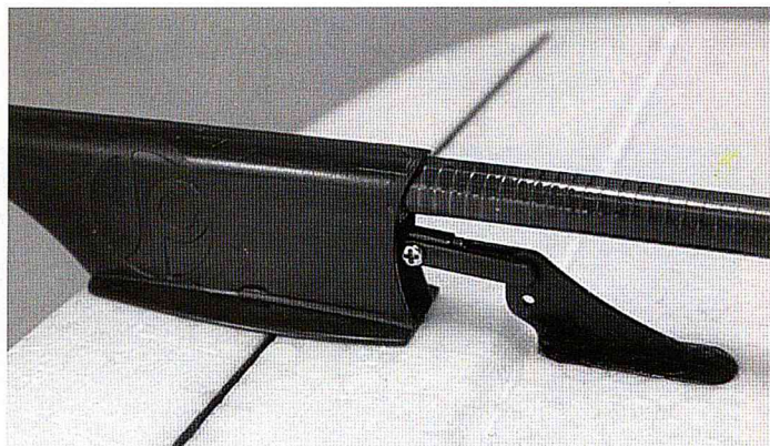
Aerodynamisch schön ausgelegte Höhenruderanlenkung
